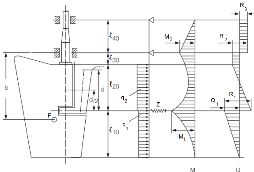
Rys. 2.2.4.4.1-1. Ster półpodwieszony z jedną elastyczną podporą
