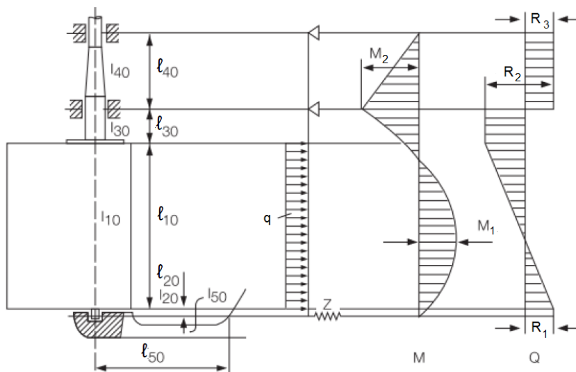
Rys. 2.2.4.2.1. Ster podparty
