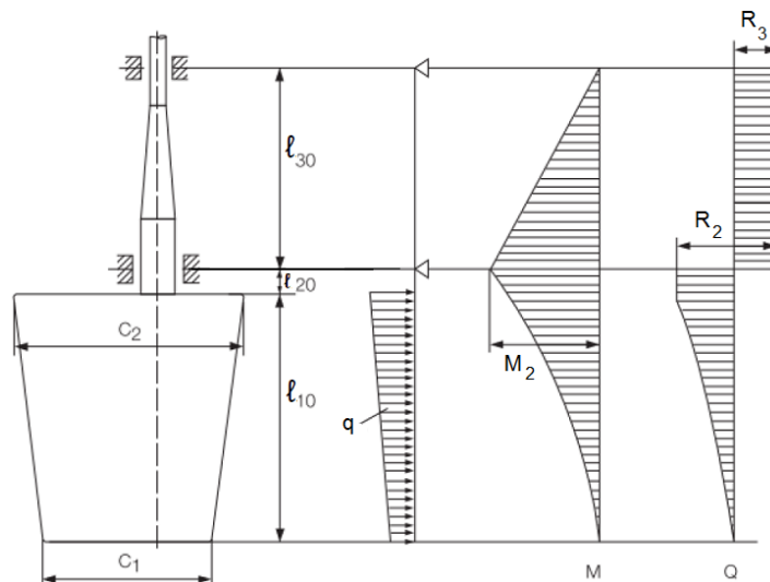
Rys. 2.2.4.3.1. Ster podwieszony bez tulei sterowej
