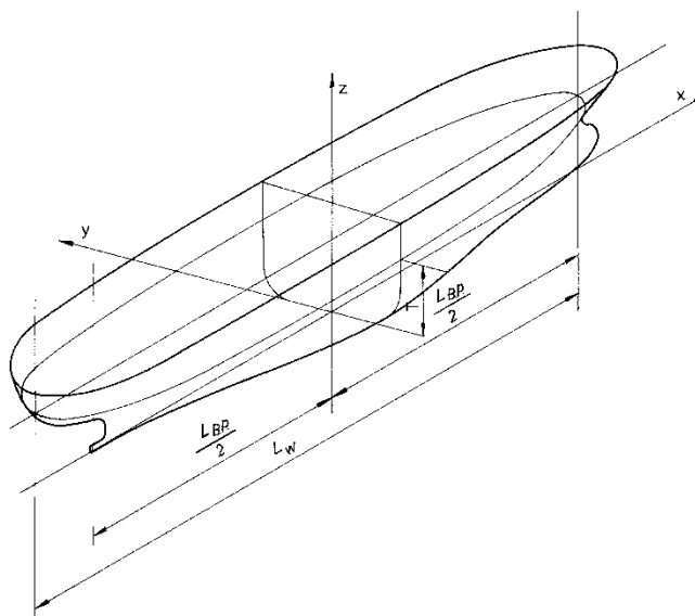
Rys. 1.2.2.1. Układ współrzędnych
