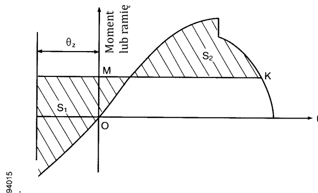
Rys. 1. Krzywa stateczności statycznej
