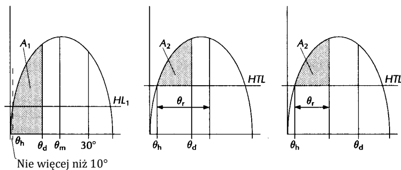
Rys. 1. Stateczność jednostki nieuszkodzonej
