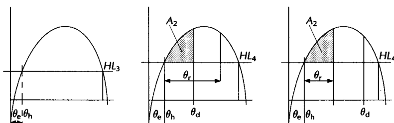
Rys. 1. Stateczność jednostki nieuszkodzonej
