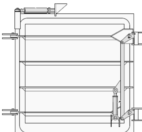
Furta do przyjmowania paliwa – typu 2, widok od wewnątrz
