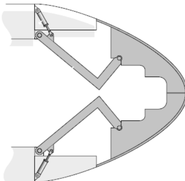
Furta dziobowa otwierana na boki – w stanie zamkniętym, widok z góry
