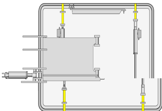
Furta do przyjmowania paliwa – typu 1, zamknięta, widok od wewnątrz
