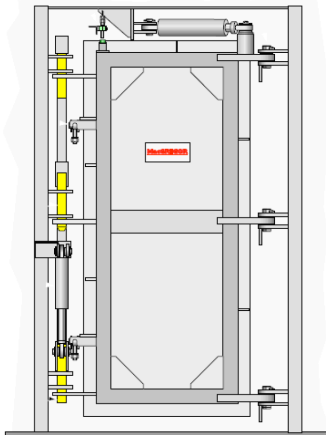
Furta do przyjmowania paliwa – w stanie zamkniętym, widok od wewnątrz
