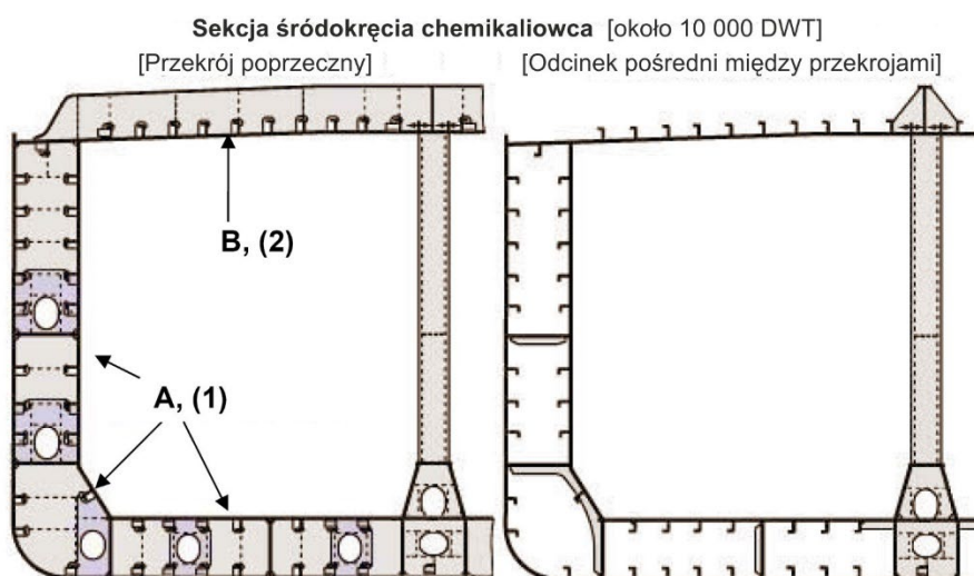
Rys. 2.1. Reprezentatywny przekrój poprzeczny chemikaliowca. Rejony A i B oraz 1 i 2.
