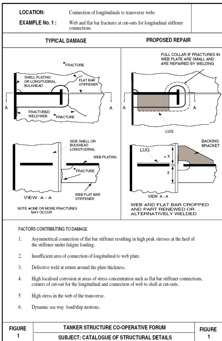
Rys. 2. Typowe uszkodzenia i przykład naprawy (reprodukcja z dokumentu związanego 1)
