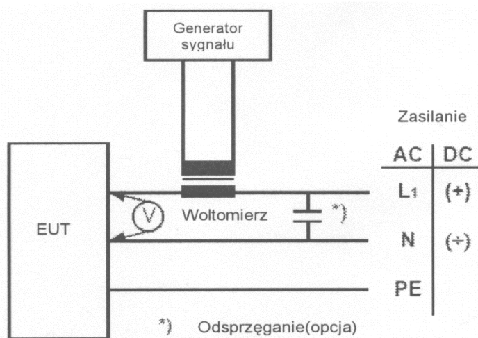
Rys. 2.19. Układ do przeprowadzenia próby zakurzzenia przewodzonego niskiej częstotliwości.
