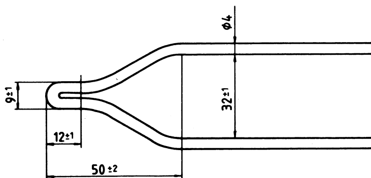
Rys. 2.25.3-1. Pętla żarowa (wymiary w mm)
