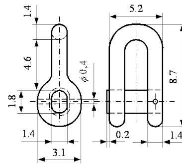
Fig. 20.3.1.1-6. End shackle
