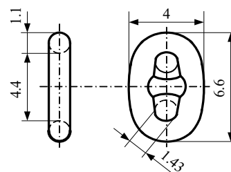
Fig. 20.3.1.1-2. Enlarged link
