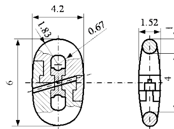
Fig. 20.3.1.1-4. Kenter shackle
