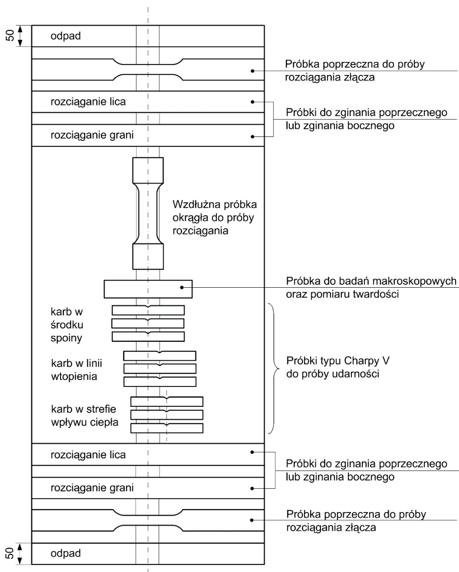
Rys. 3. Rozmieszczenie próbek do badań niszczących złącza próbnego ze spoiną czołową
