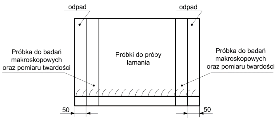
Rys. 4. Rozmieszczenie próbek do badań niszczących złącza próbnego ze spoiną pachwinową
