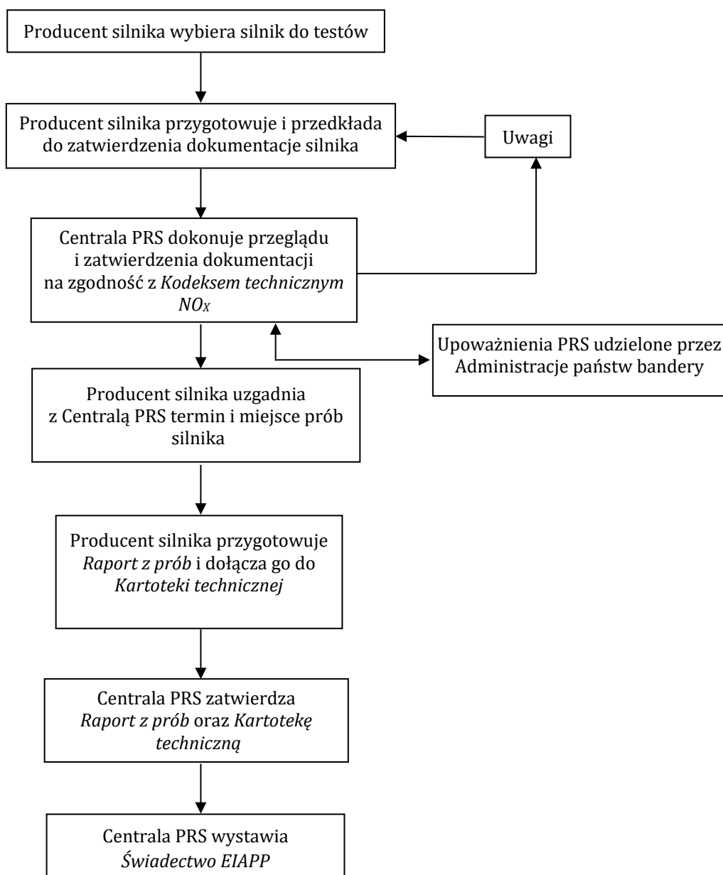
Rys. 1. Schemat blokowy – Przedwstępny przegląd certyfikacyjny u producenta silnika
