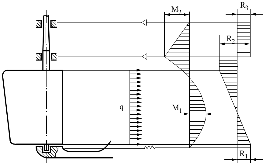
Rys. 2.2.2.1. Obciążenia, momenty gnące i siły tnące w sterze podpartym
