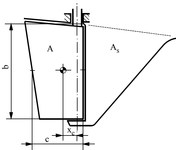
Rys. 2.2.3.3. Ster podparty z dużym statecznikiem ( A/A_s < 2 )
