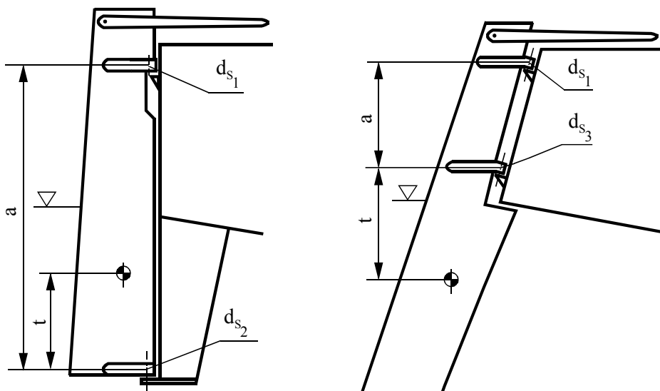
Rys. 2.5.2. Stery pawężowe
