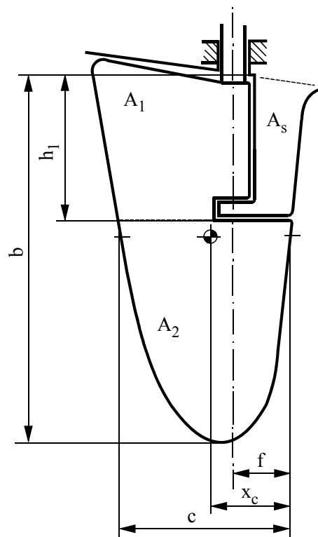
Rys. 2.2.3.4. Ster podwieszony
