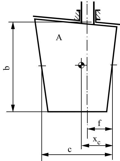
Rys. 2.2.3.4. Ster podwieszony
